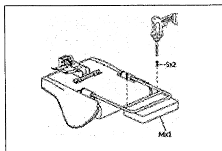
7. Fixed footrest 6*30:2
